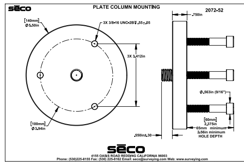
2072-52 — Column Plate
